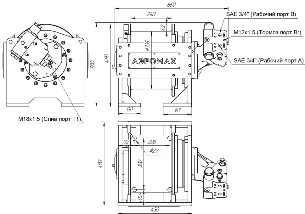
Рис.1 – Габаритные и присоединительные размеры изделия
