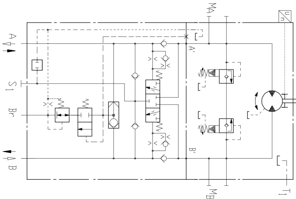
Рис.2 – Схема гидравлическая принципиальная А, В – рабочие порты, Вr- тормоз, Т1-слив.
